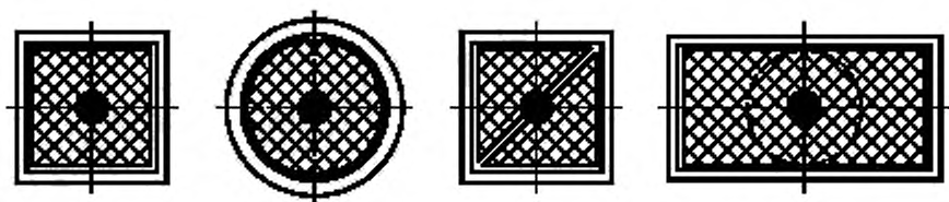
Рисунок Е.1 — Расположение пуансона на люках и (или) дождеприемниках при испытаниях на механическую прочность
