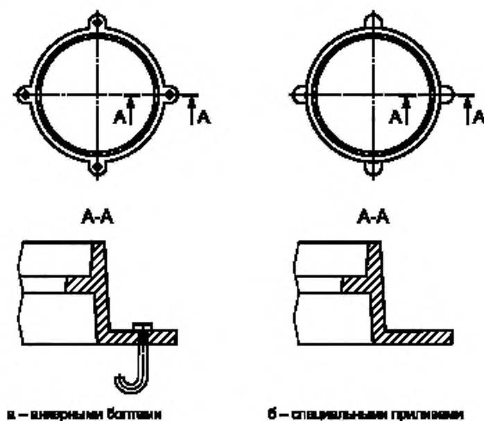
Рисунок А.4 — Усиленная заделка корпуса
