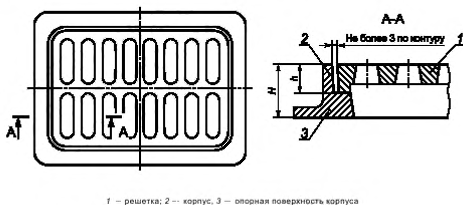
Рисунок В.1 — Дождеприемник с равной шириной опорной части корпуса
