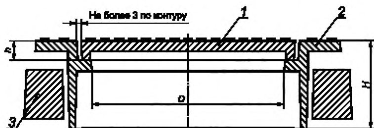
Рисунок А.7 — Люк с самонивелирующим (плавающим) корпусом
