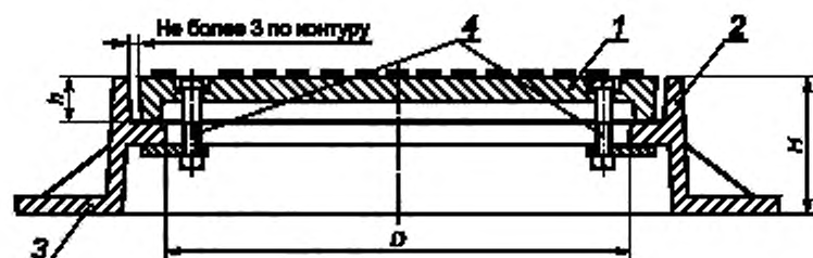
1 — крышка; 2 — корпус; 3 — опорная поверхность корпуса; 4 — замковое устройство
