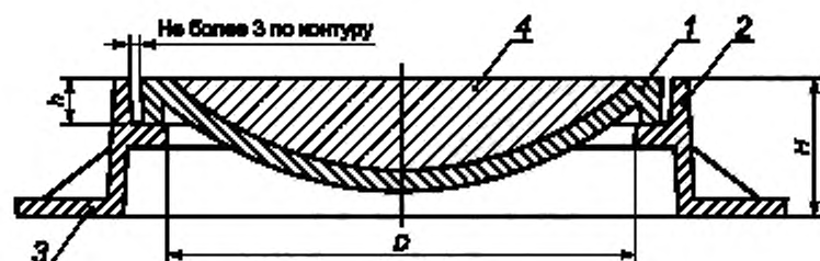
1 — крышка; 2 — корпус; 3 — опорная поверхность корпуса; 4 — бетон
