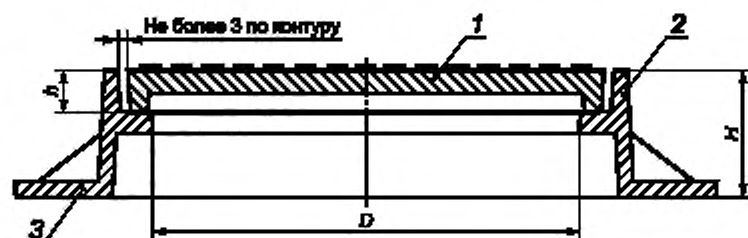
1 — крышка; 2 — корпус; 3 — опорная поверхность корпуса
